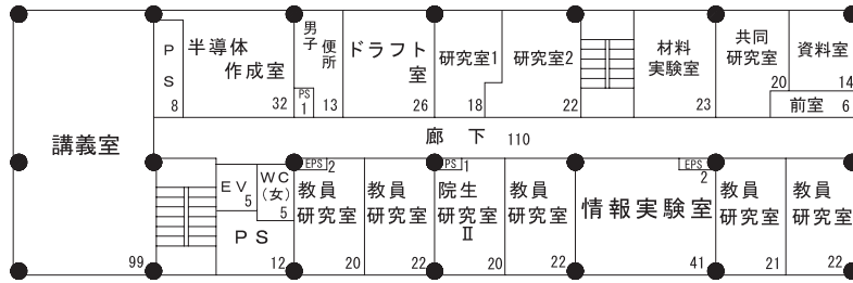
6階平面図
