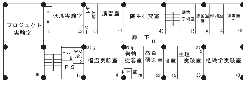
5階平面図
